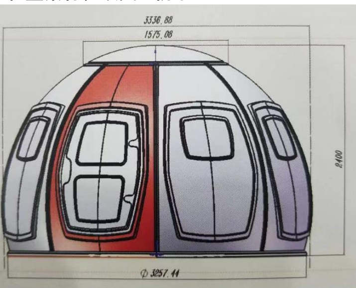
トップサン カットカバー
